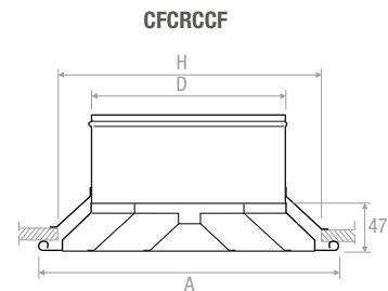
CF Collarino di fissaggio Fixing ring
